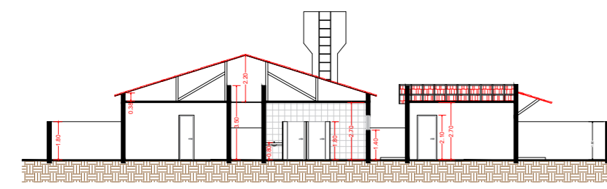
CORTE A-A
