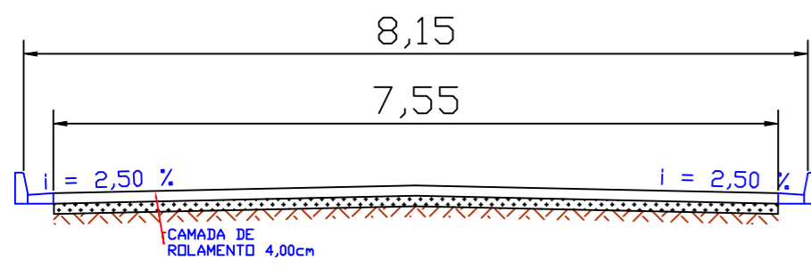
SEÇÃO TRANSVERSAL S/ ESC.
