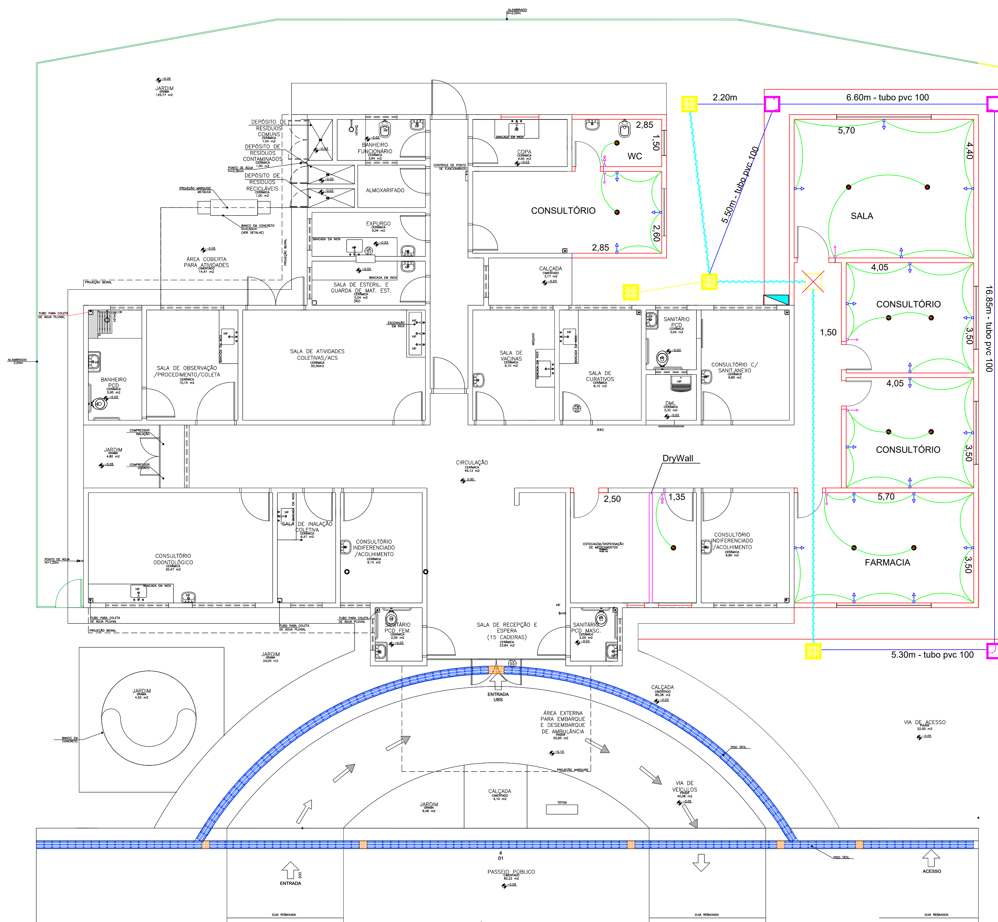
Planta Baixa - Ampliação - Projeto Elétrico - Iluminação e esgoto ESCALA 1:100
