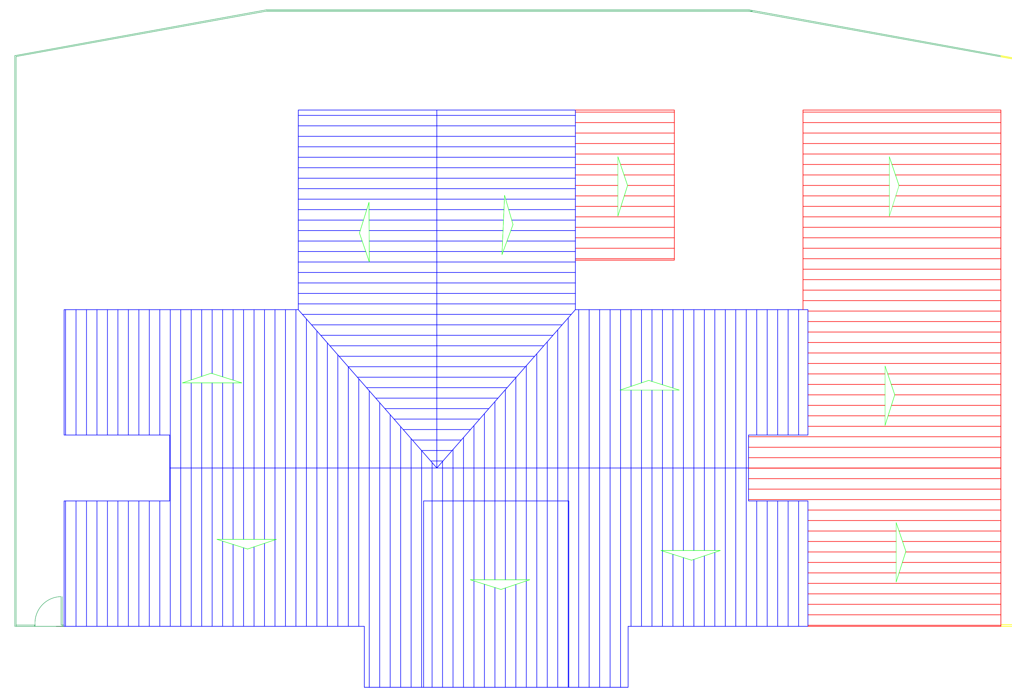
Cobertura ESCALA 1:100
