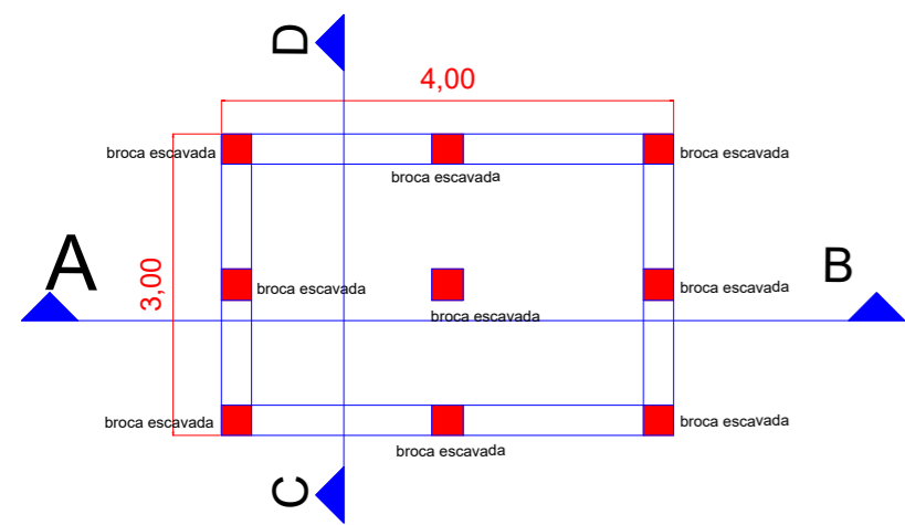
Planta baixa Caixa de captação
