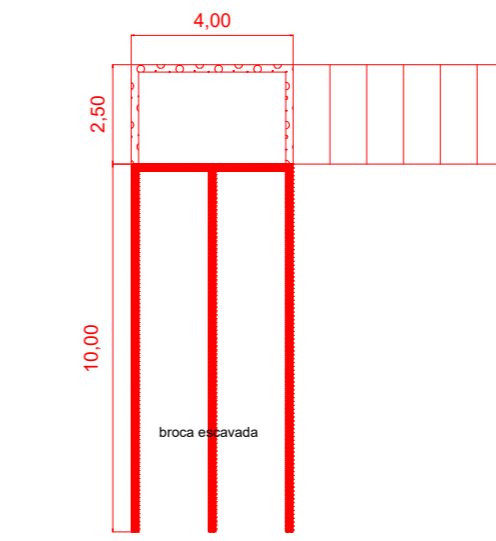
CORTE A-B
