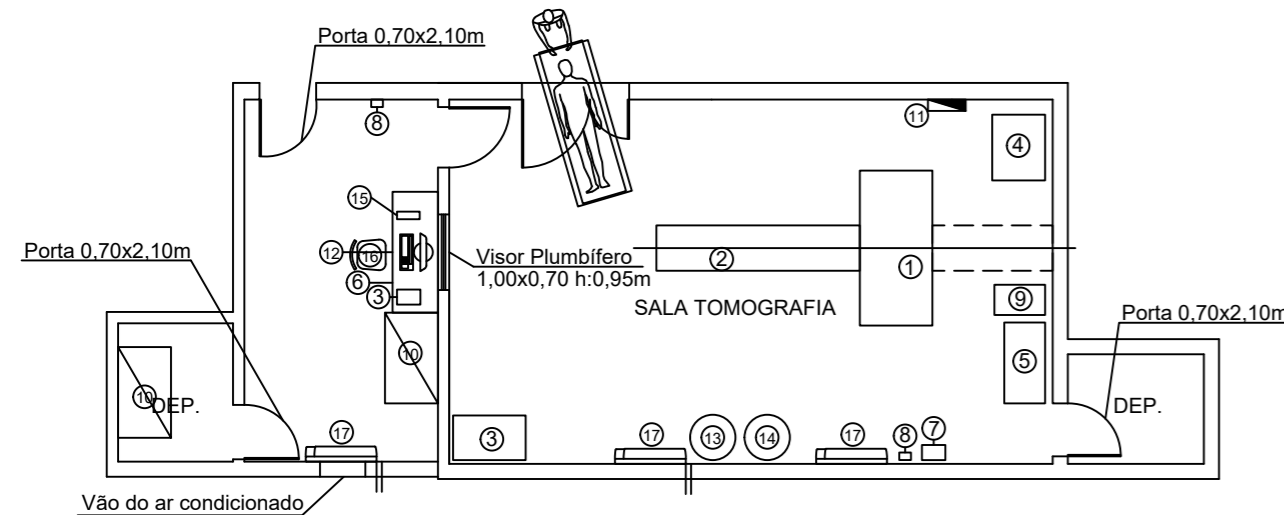
PLANTA MOBILIÁRIO Esc.: 1:100
