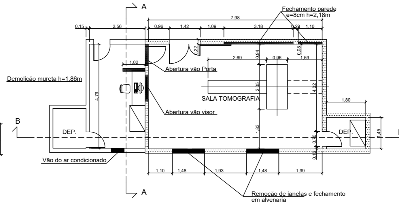
PLANTA BAIXA Esc.: 1:100
