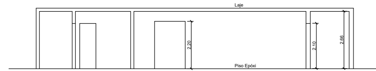
CORTE B-B Esc.: 1:100
