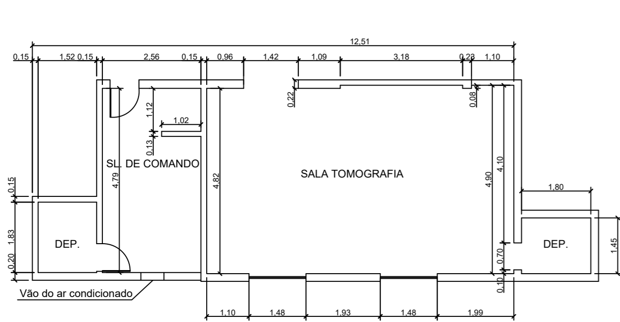
PLANTA BAIXA - Situação atual Esc.: 1:100
