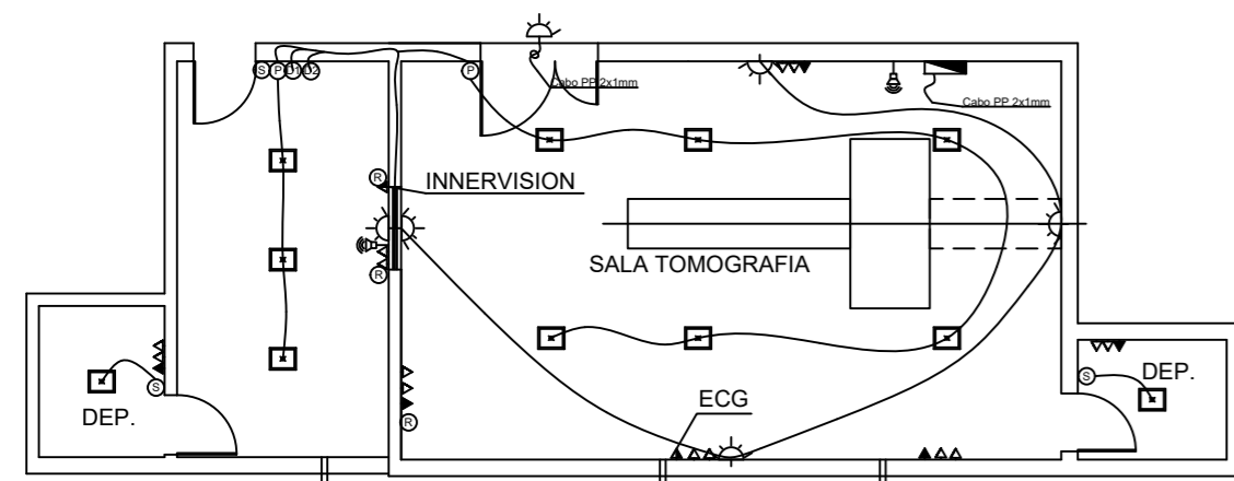
PLANTA DE ELÉTRICA Esc.: 1:100
