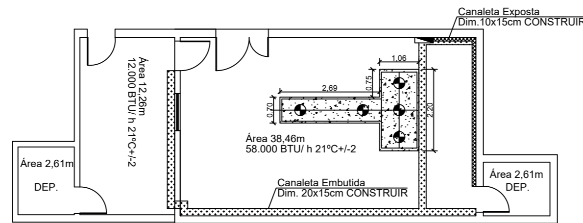
PLANTA PISO Esc.: 1:100
