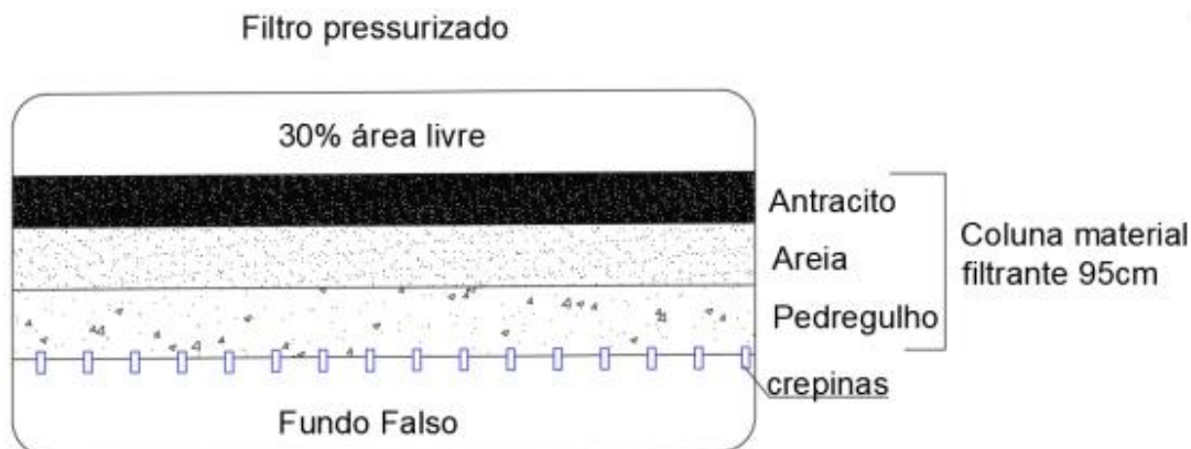
Figura 01 – Filtro
