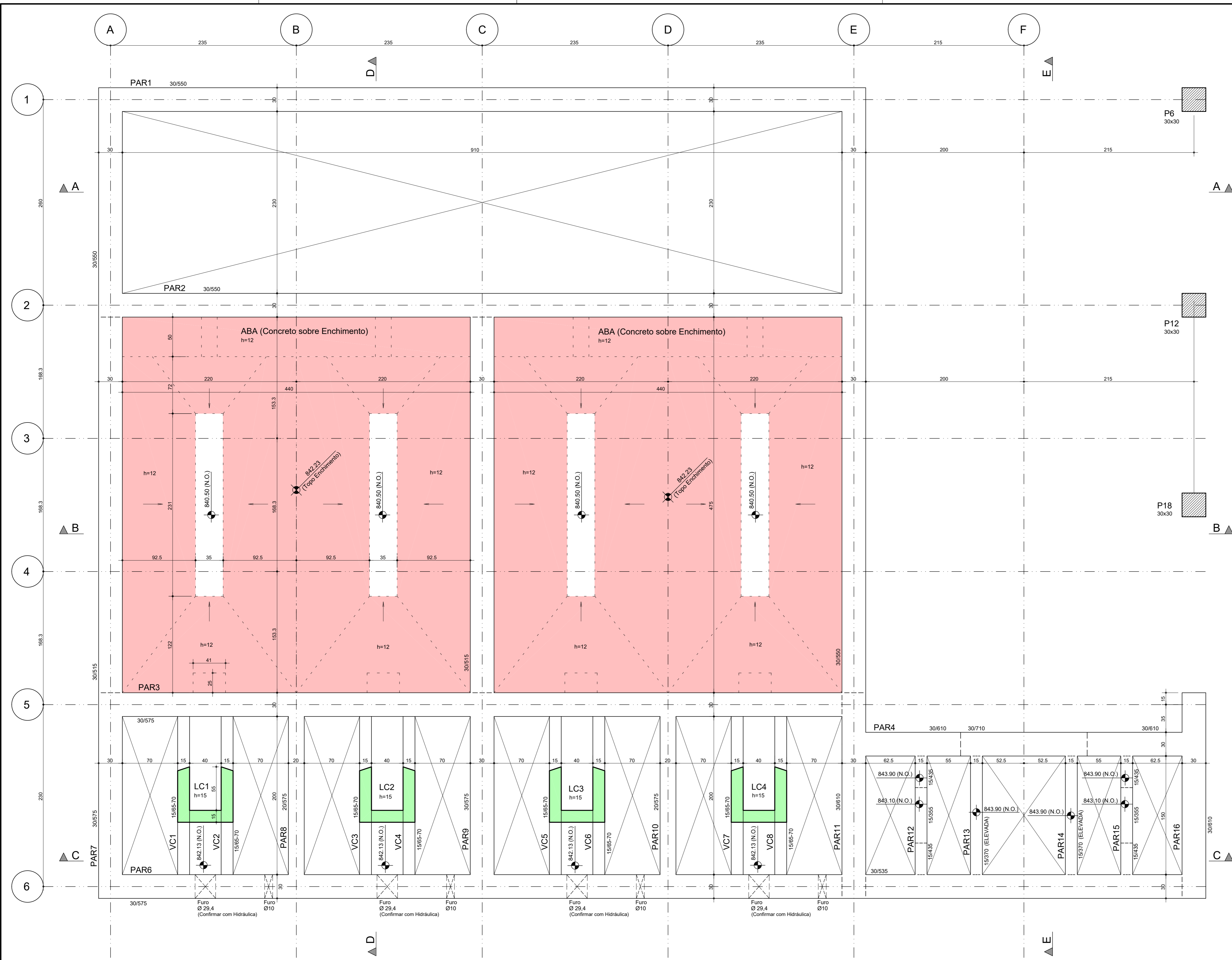
FORMA - NÍVEL 842.13 1:25
