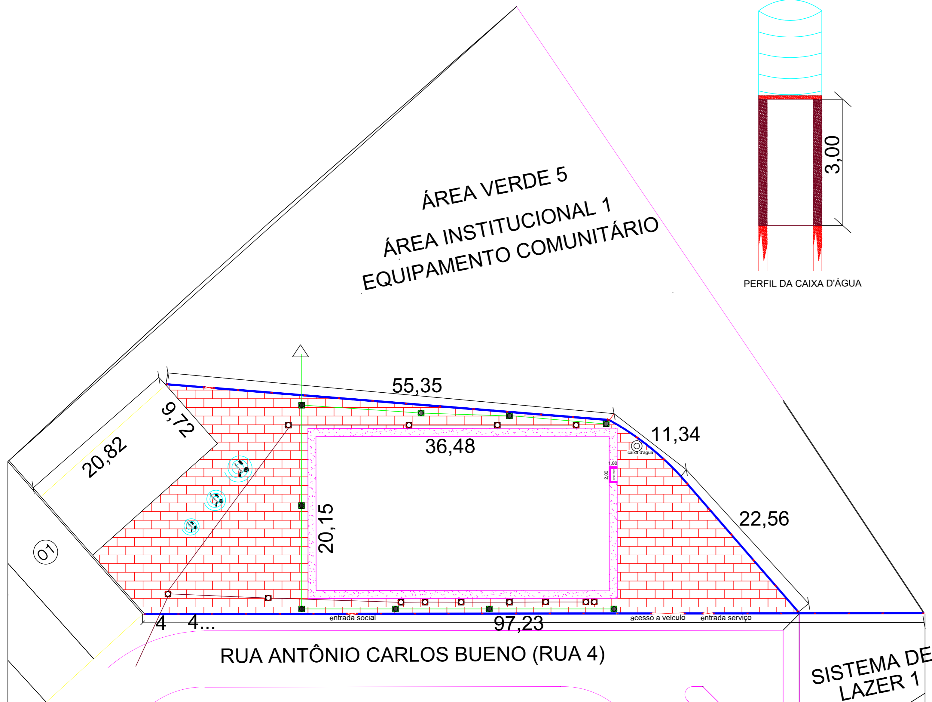
Planta baixa dos PV's Tubulação e Pisos
