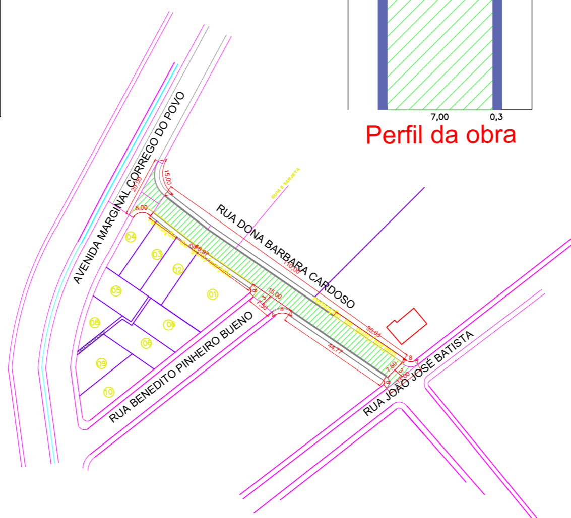
Pavimentação tipo CBUQ
