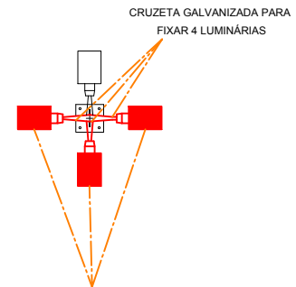
LUMINÁRIA DE LED RETÂNGULAR PARA POSTE EFICIÊNCIA MÍNIMA 113 lm/W
